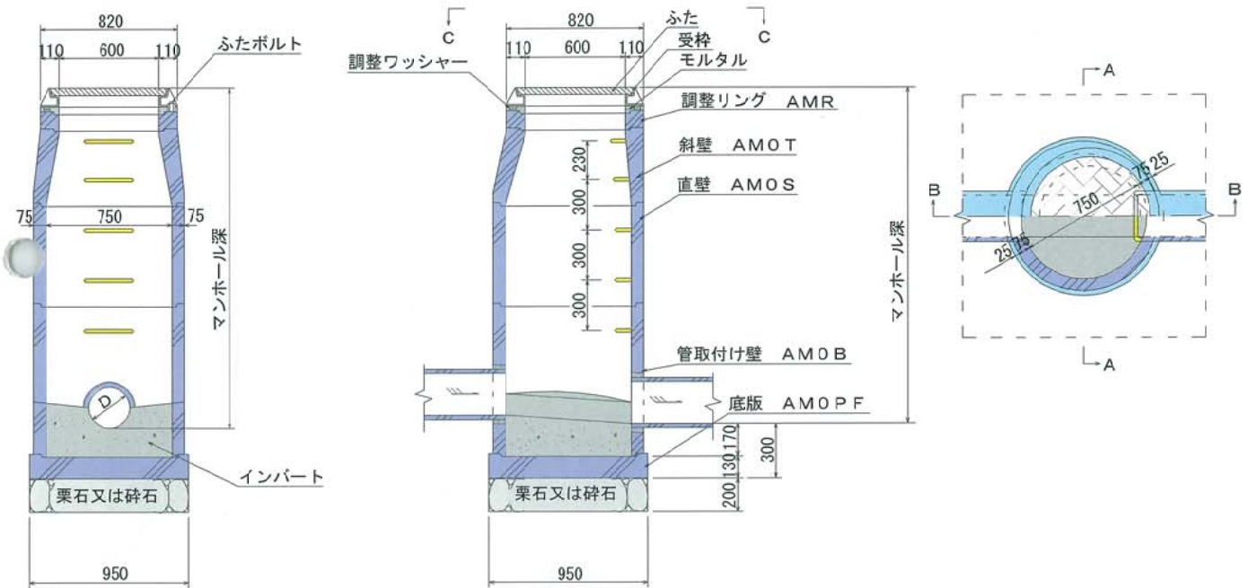
■A-A断面図
