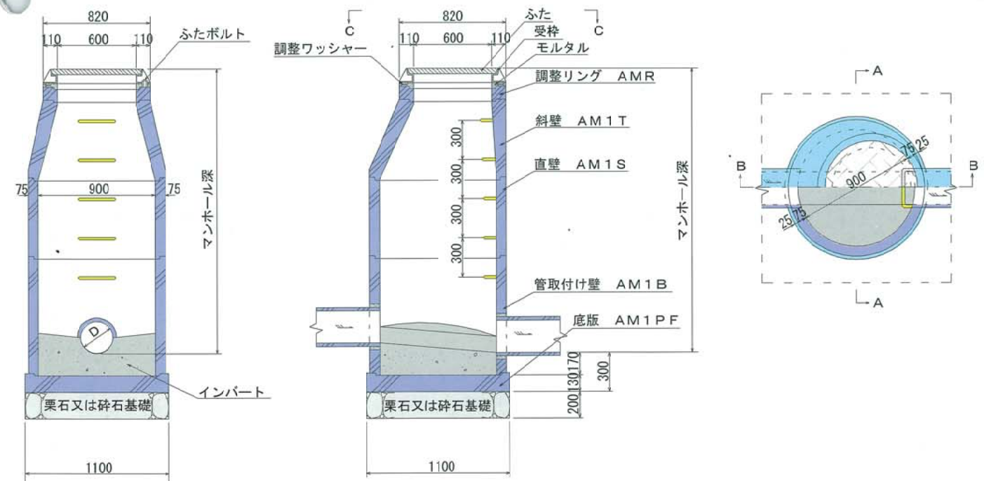
■A-A断面図
