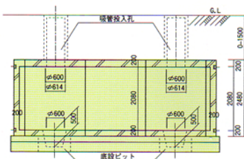
側面図
