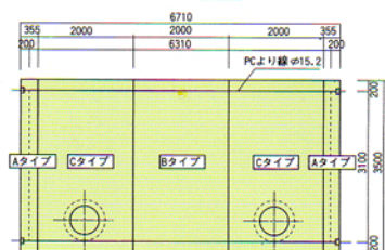
平面図
