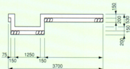
D-D断面図
