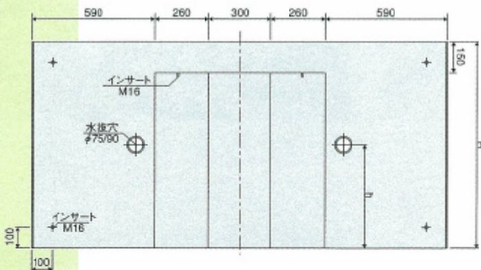
背面図
