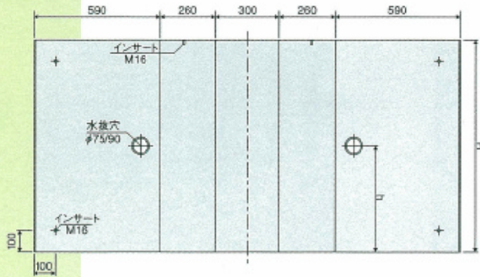
背面図
