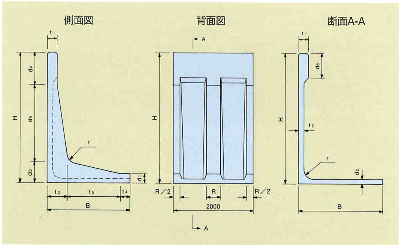
規格寸法表
