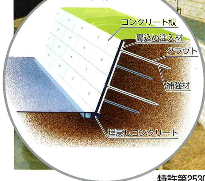
一般構造図
