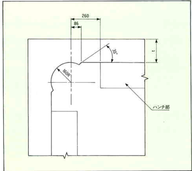
隅部において工場製品を使用する場合
