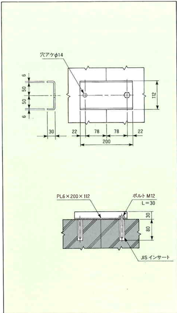
隅部において工場製品を使用する場合
